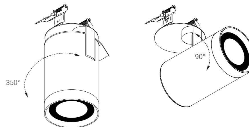
TERES EXTE RECESSED
